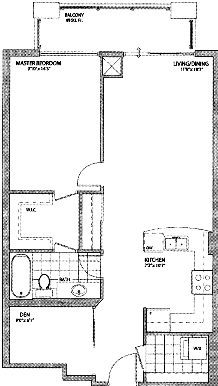
TYPE F1 ONE BEDROOM + ONE BATH + DEN 793 SQ. FT.
